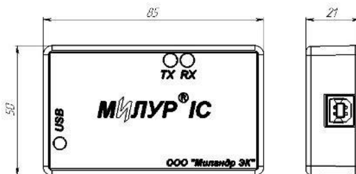
Рисунок 2 - Габаритные и установочные размеры МИЛУР IC UR-Z/P
