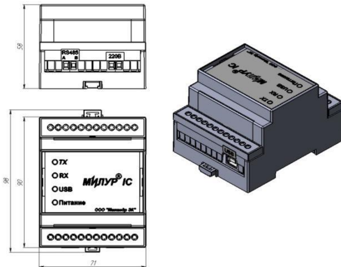
Рисунок 2 - Габаритные и установочные размеры МИЛУР IC UR-Z/P
