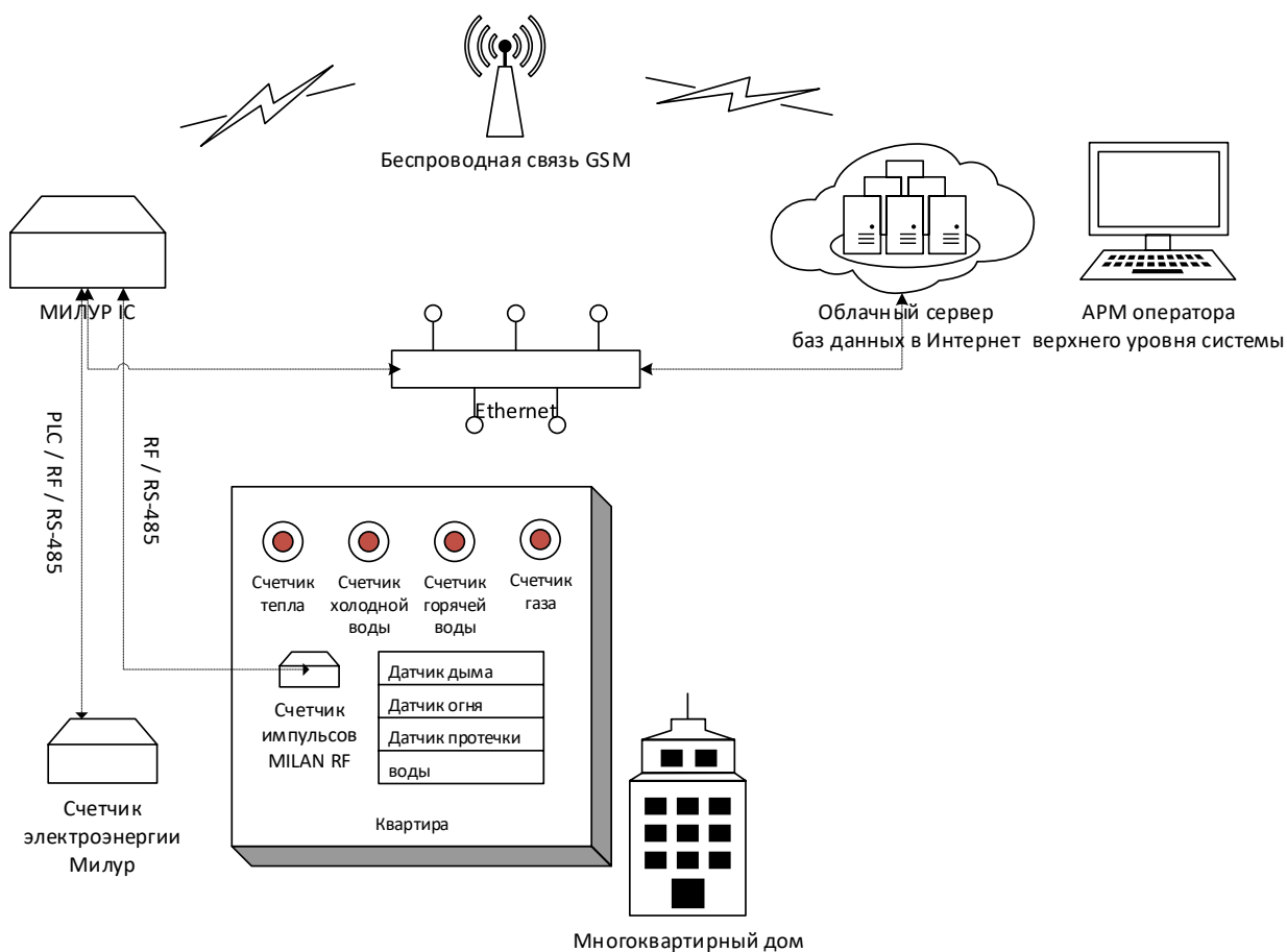
Рисунок 1 – Примерная схема системы многоквартирного дома
