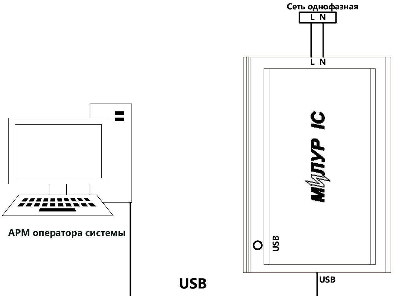
Рисунок 8 – Подключение МИЛУР IC U-P
