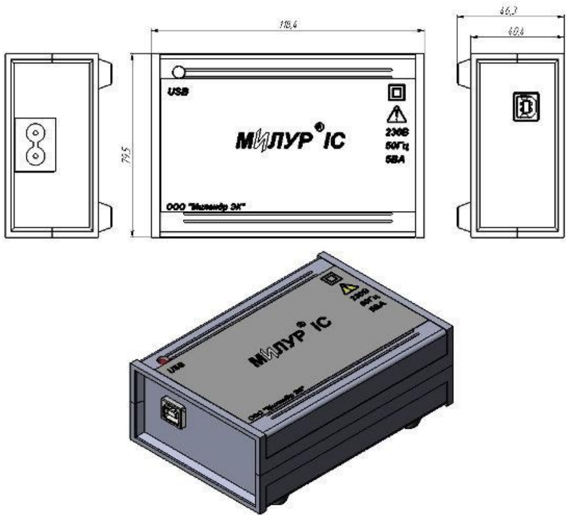
Рисунок 4 - Габаритные и установочные размеры МИЛУР IC U-P, R-P, R-Z
