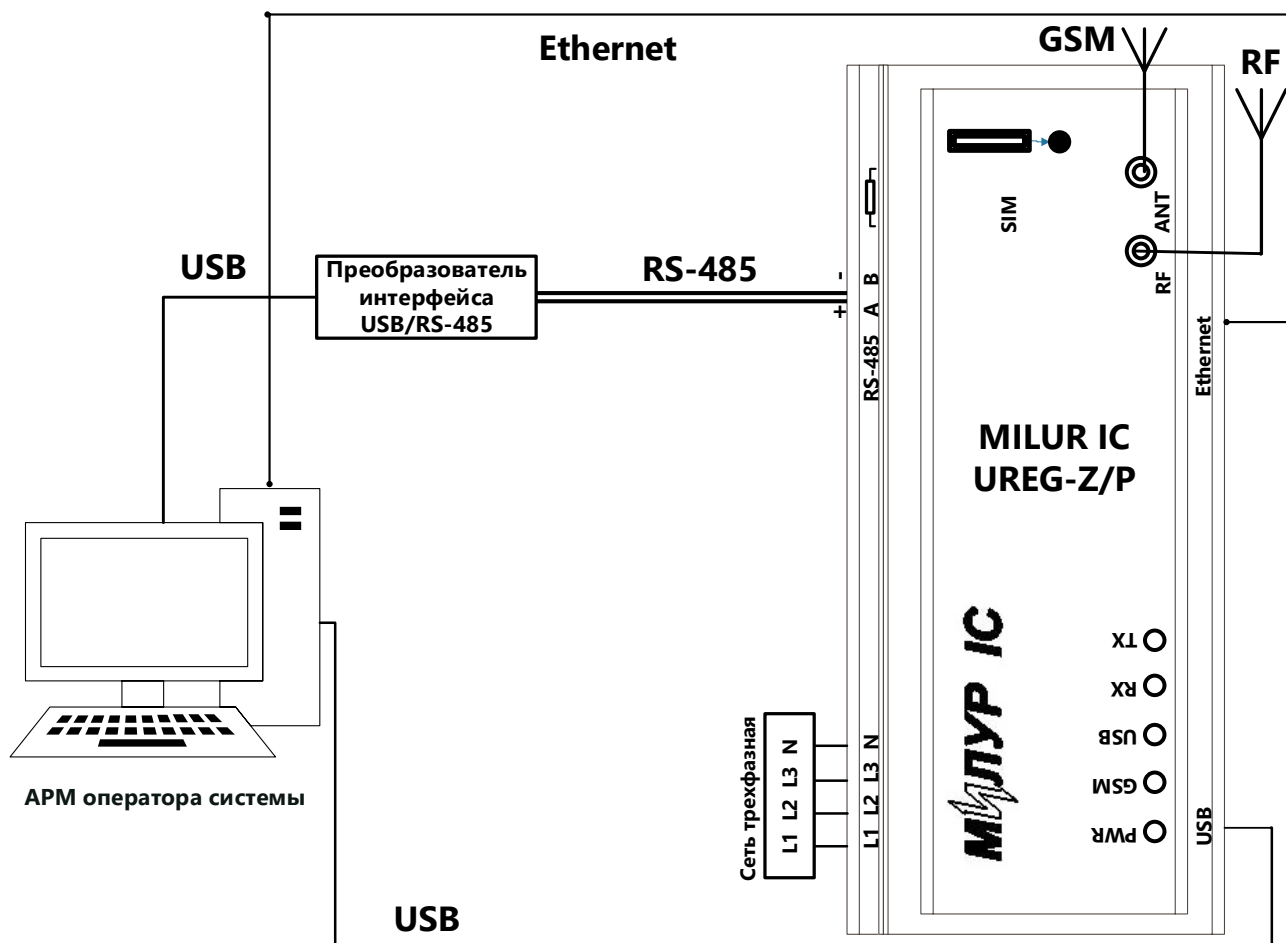
Рисунок 9 – Подключение МИЛУР IC UREG-Z/P (допускается подключение к изделию как одного, так и нескольких интерфейсов)
