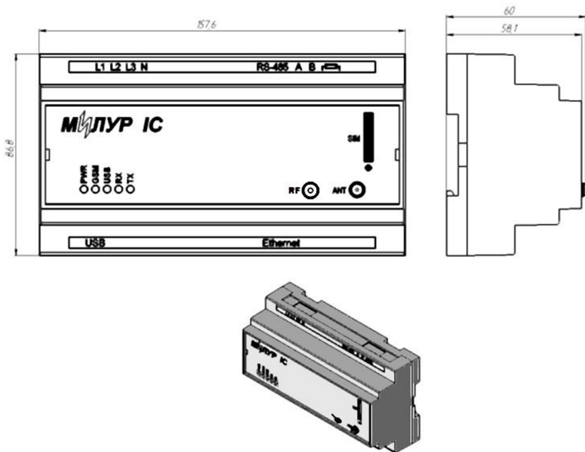
Рисунок 5 - Габаритные и установочные размеры МИЈУР IC UREG-Z/P, UREG-P, UREG—Z, URE-Z/P, URE-P, URE-Z
