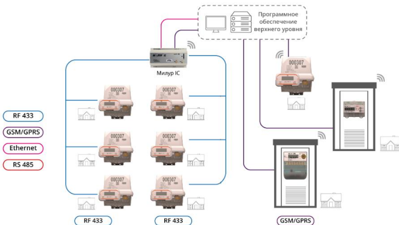
Рисунок 20 – двухуровневая архитектура ИСУЭЭ в частном секторе
