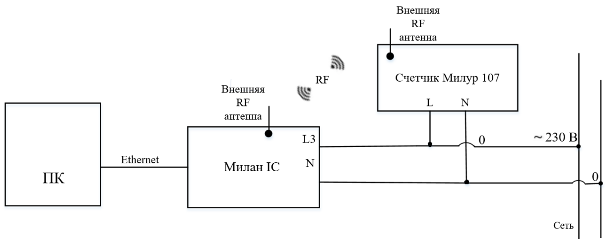
Рисунок Е.5 – Схема подключения счетчика к ПК через интерфейс RF868
