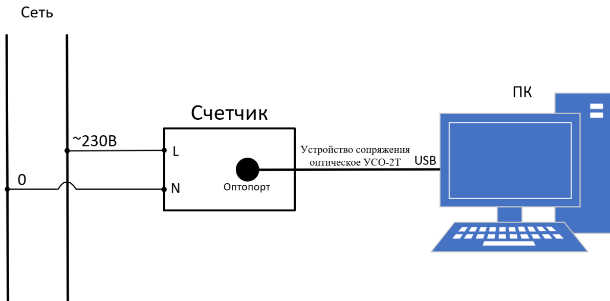
Рисунок 24 – Подключение счетчика к ПК через оптопорт
