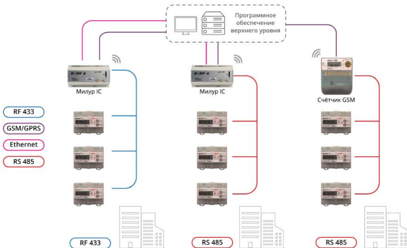
Рисунок 22 – двухуровневая архитектура ИСУЭЭ в МКД
