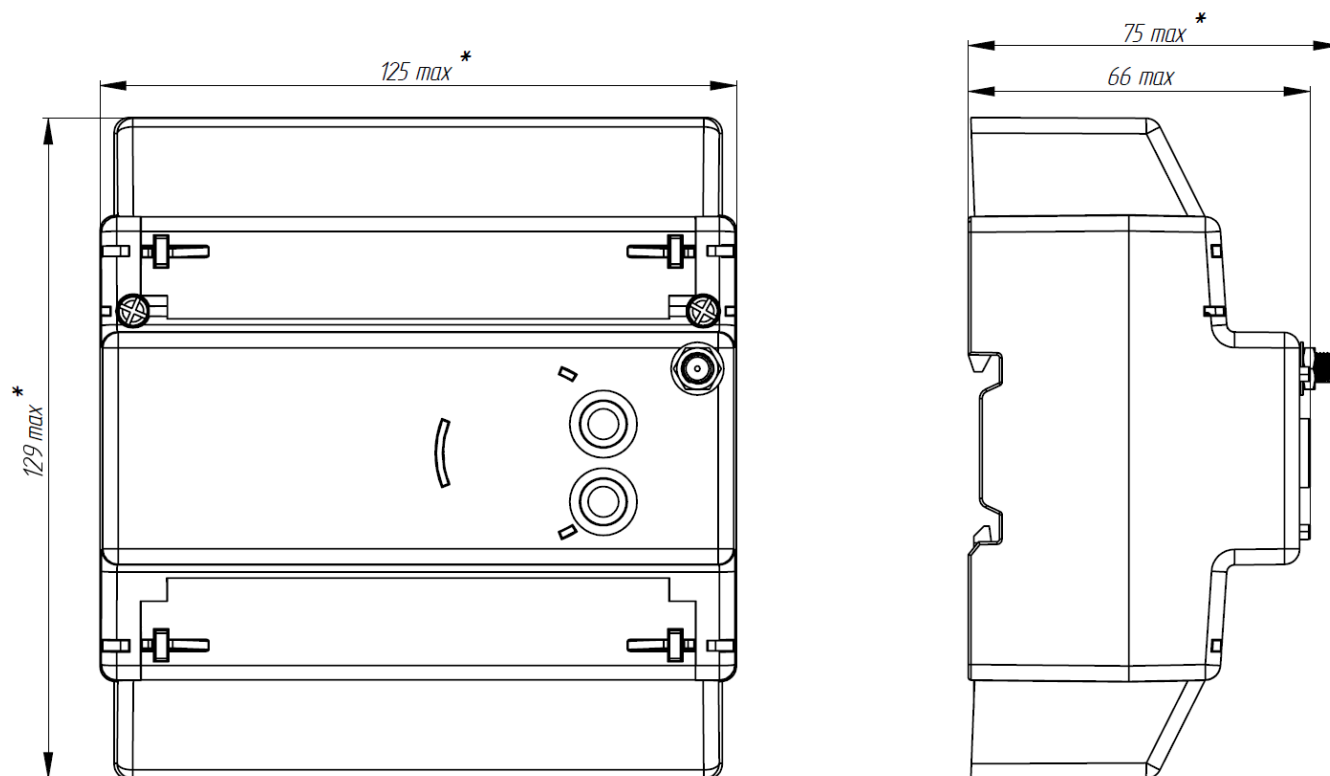
Рисунок Б.2 – Корпус 7mTH35 со стандартными клеммными крышками (антенна показана условно и не входит в комплект поставки счетчика, * габаритные размеры)
