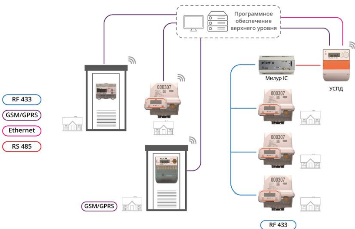
Рисунок 21 – трехуровневая архитектура ИСУЭЭ с применением УСПД в частном секторе
