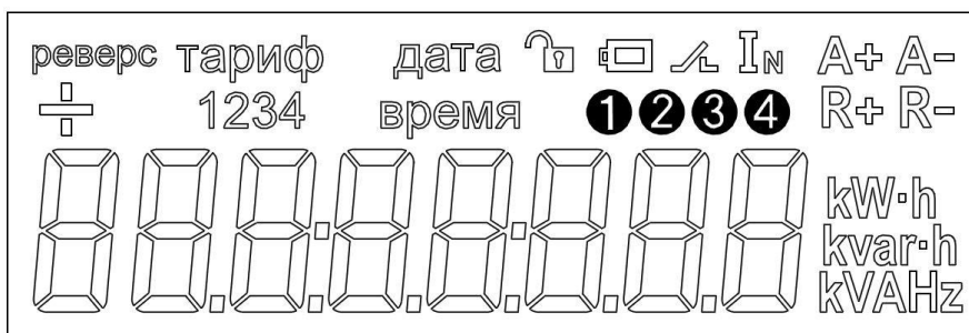
Рисунок 8 - Общий вид ЖКИ счетчиков в корпусе 7mTH35
