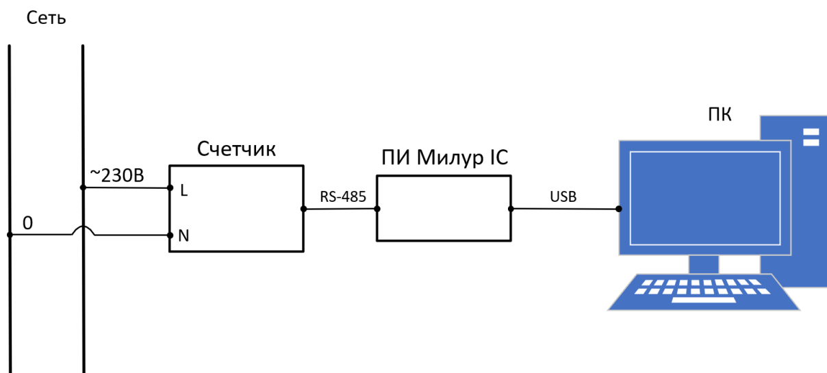
Рисунок 25 – Подключение счетчика к ПК через интерфейс RS-485 с помощью преобразователя интерфейсов Милур IC
