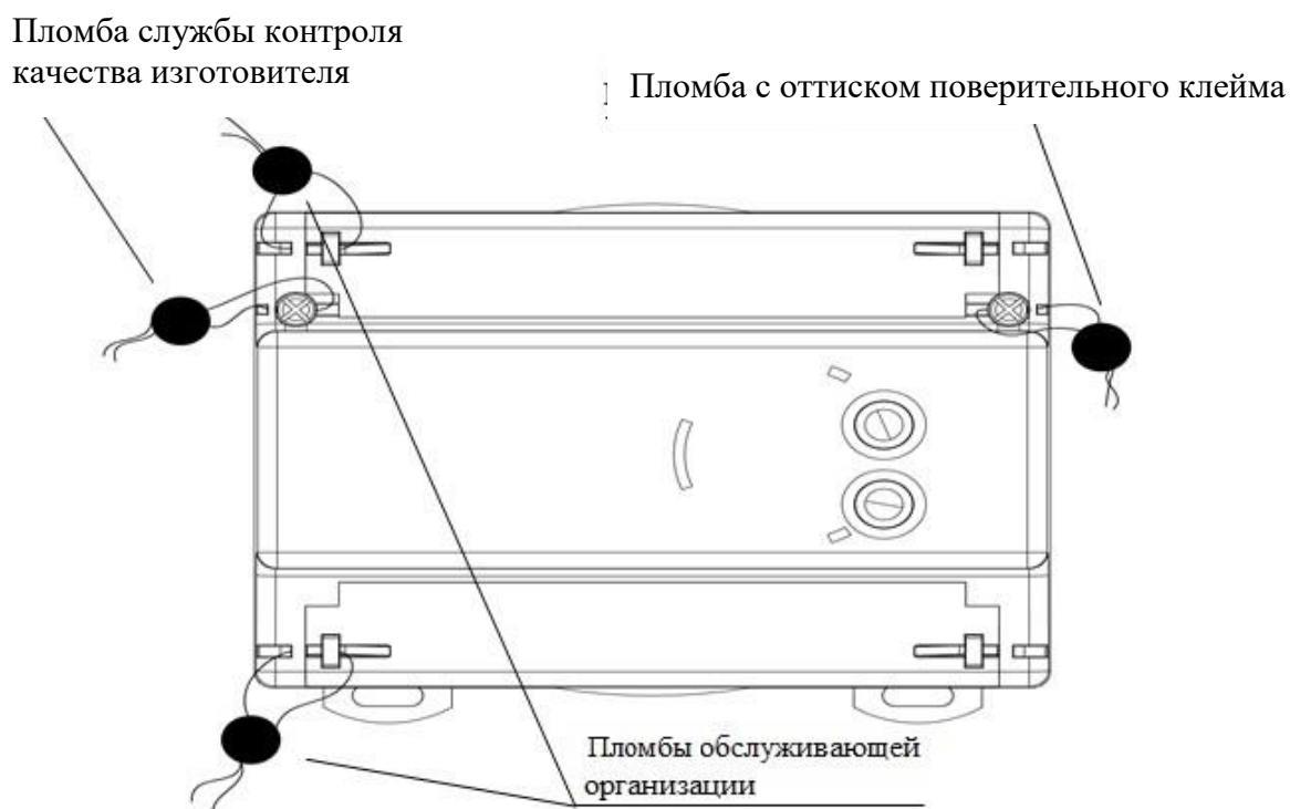
Рисунок 5 - Схема пломбировки для счетчиков в корпусе 7мТН35
