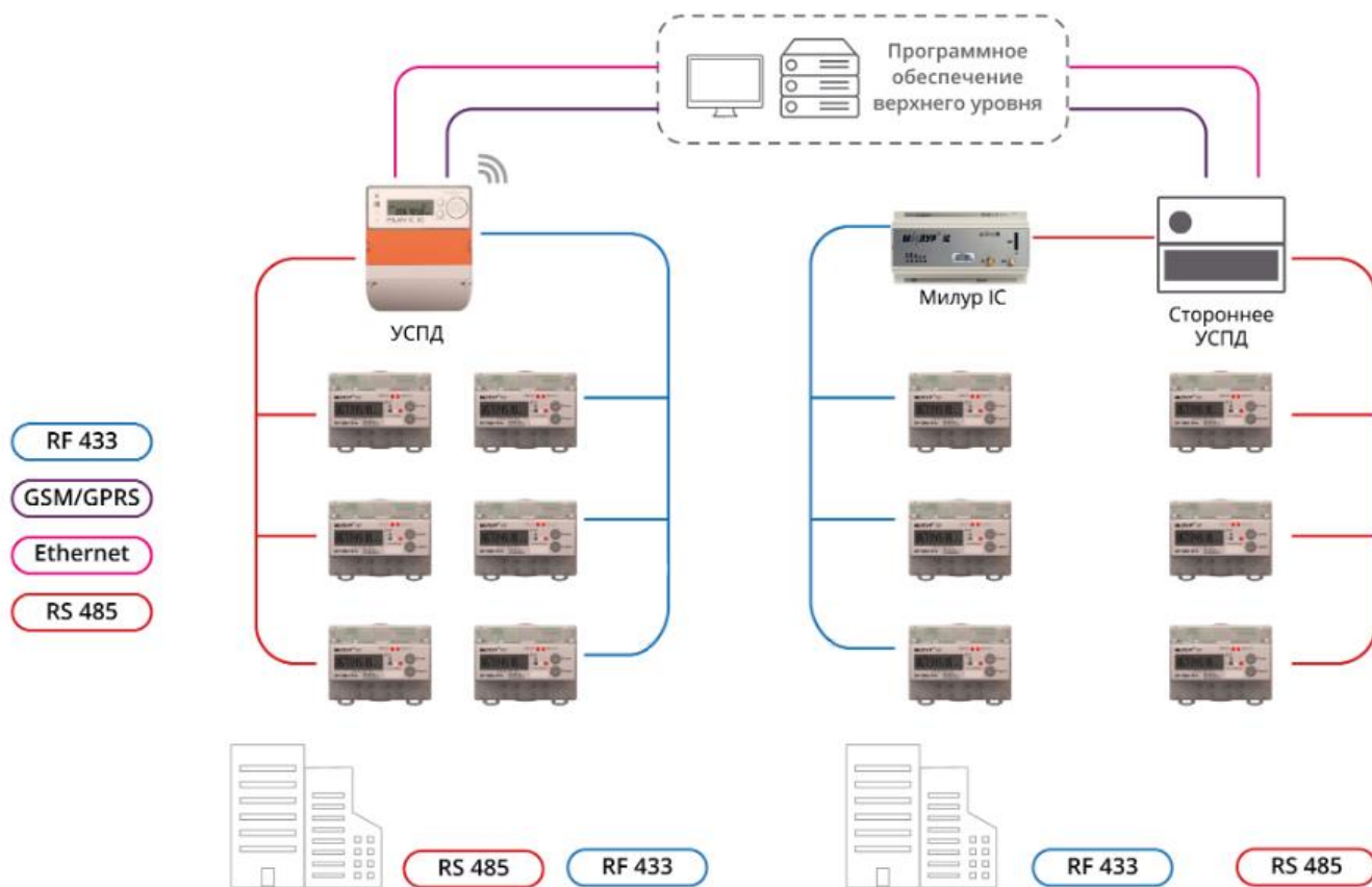
Рисунок 23 – трехуровневая архитектура ИСУЭЭ с применением УСПД в МКД
